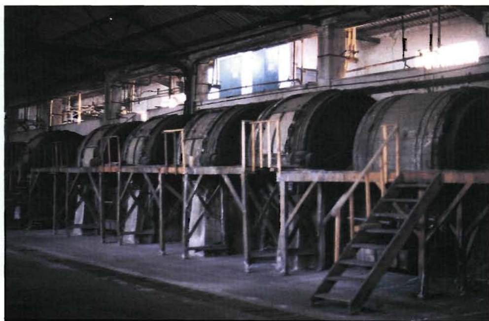
Οι βαρέλες, όπου γινόταν η κατεργασία των δευμάτων με ασβέστη και κανστική σόδα (φωτό Γ. Ιορδάνου).
