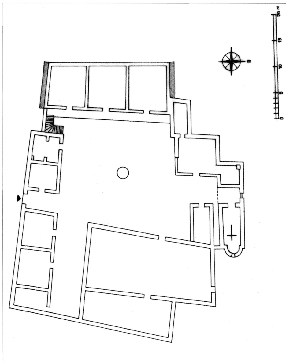
Κάτοψη του κτιριακού συγκροτήματος του μετοχίου της Μονής Πάτμου στο λόφο του Παλαιόκαστρου, εντός του αρχαιολογικού χώρου των Απτέρων (σχέδιο Ιωάννα Τραχανά).
