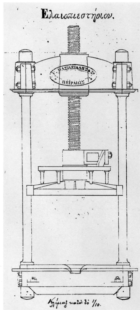
9. Σχέδιο (όψη) του ελαιοπιεστηρίου της εικ. 8, που συνόδευε επιστολή του μηχανουργείου Βασιλειάδη προς τον Αθαν. Δουρούτη, 19.1.1867. Στο κάτω μέρος: «Κλίμαξ κατά το 1/10» (Αρχείο Χ. Ζιούλα, διαστ. σχεδίου 22Χ10,5 εκατοστά).
