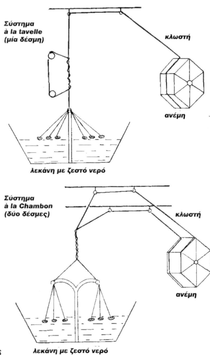
6. Σχηματική παράσταση των δύο συστημάτων αναπήνισης (από: I.Brossard, Technologie des textiles , Παρίσι 1977, σ. 91).
