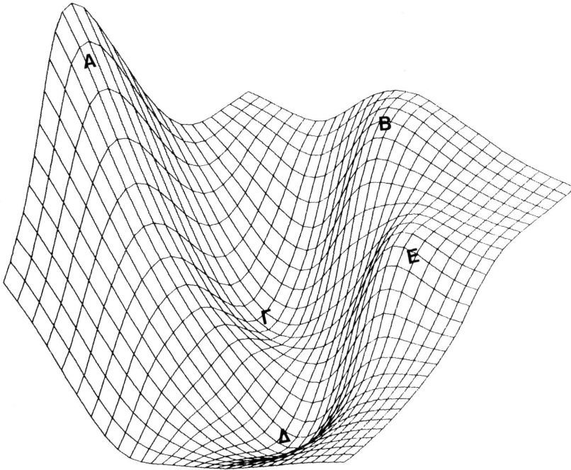
Σχήμα 3: Τρισδιάστατη απεικόνιση των ομάδων των μεταβλητών. Η θέση της κάθε μεταβλητής καθορίζεται από τις συντεταγμένες της στους 3 πρώτους παραγοντικούς άξονες. Οι ομάδες A, B, Γ, Δ και E αντιστοιχούν στις ομάδες του σχήματος 1.
