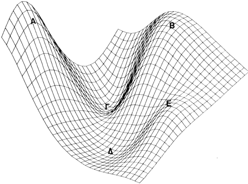
Σχήμα 2: Τρισδιάστατη απεικόνιση των ομάδων των βιβλίων. Η θέση του κάθε βιβλίου-σημείου καθορίζεται από τις συντεταγμένες του στους 3 πρώτους παραγοντικούς άξονες. Οι ομάδες A, B, Γ, Δ και E αντιστοιχούν στις ομάδες του σχήματος 1.
