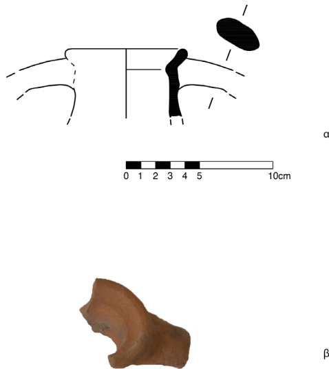
Εικ. 3α-β. Αμφορέας τύπου Hayes 38.
