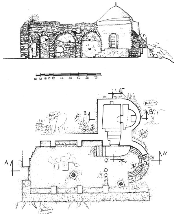
Εικ. 2. Λακωνία, όρος Μαλέας. Ο ναός του Αγίου Γεωργίου, κάτοψη.
