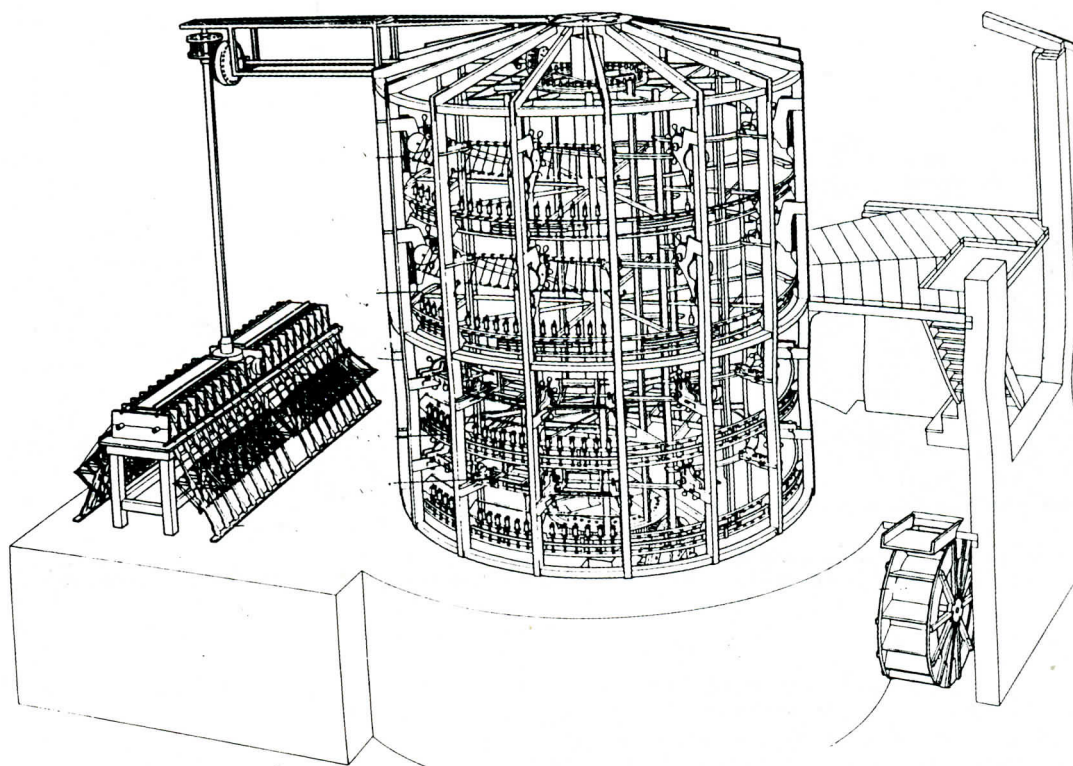
Σχέδιο του υδροκίνητου μύλου του μεταξίου από το μουσείο Aldini - Valeriani στη Μπολόνια, περ. Scuolaofficina n.1-3, 1986.
