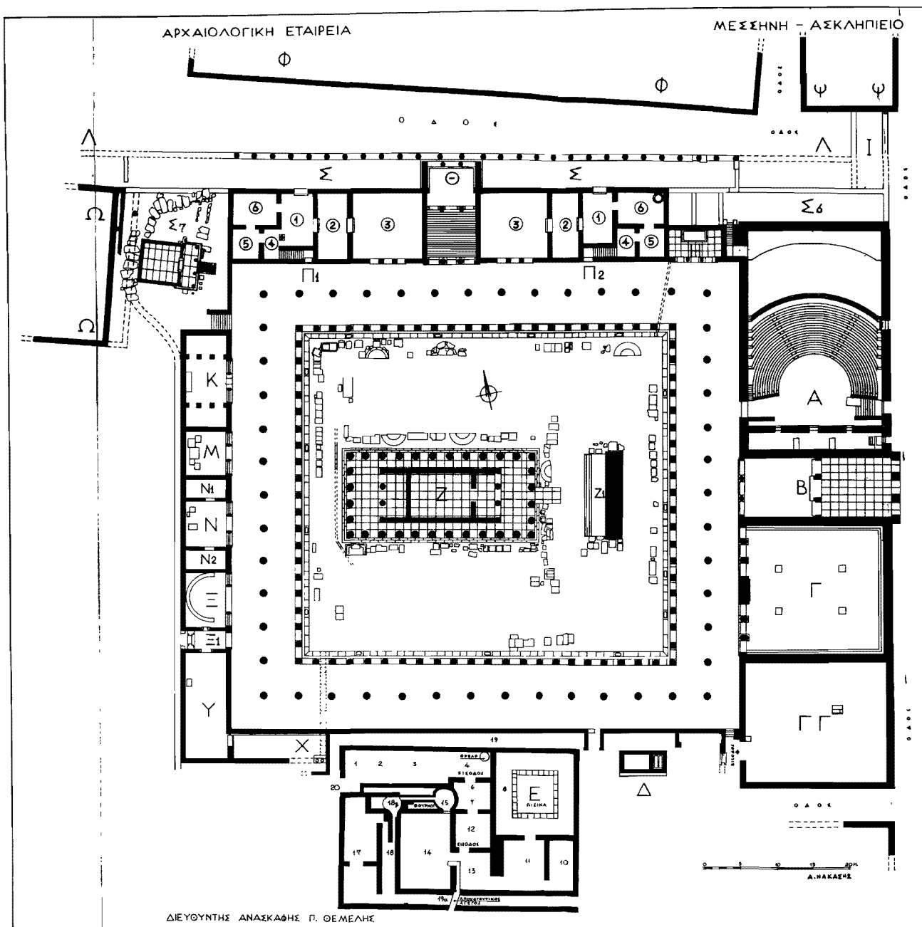
Εικ. 2. Μεσσήνη. Κάτοψη του οικοδομικού συγκροτήματος του Ασκληπείου σε αναπαράσταση (Π. ΘΕΜΕΛΗΣ, ΠΑΕ).
