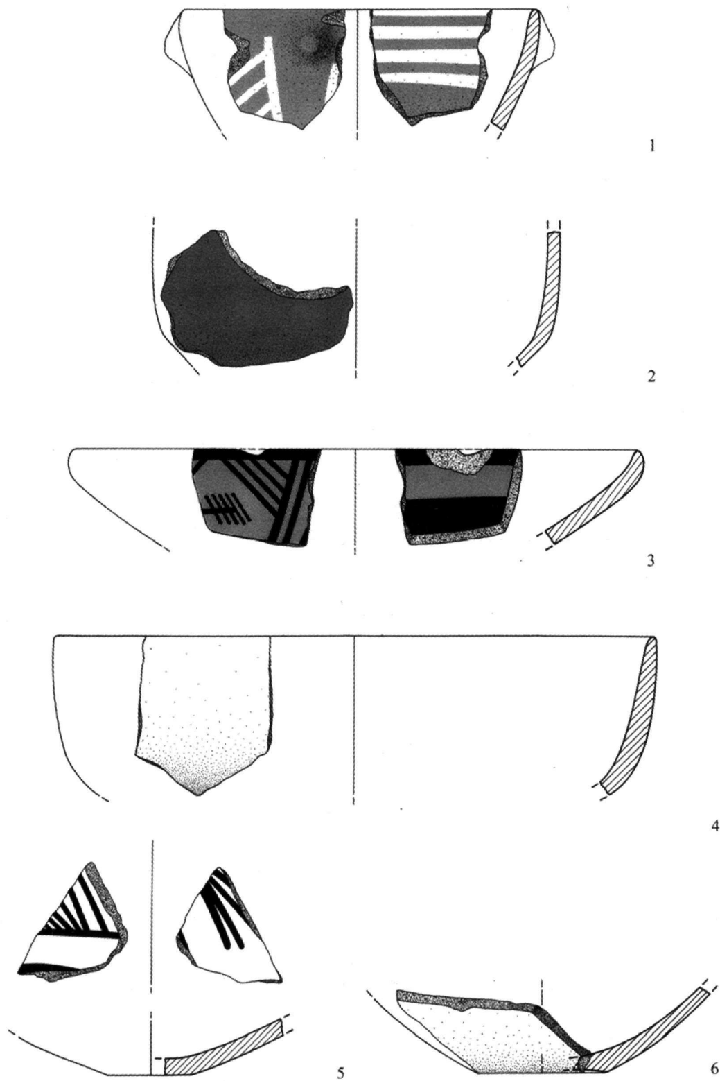
Πίνακας II.4: 1.3.5. Γραπτή, 2.4.6. Μονόχρωμη κεραμική. Στρώμα (3)-4. Κλίμακα 1:2
