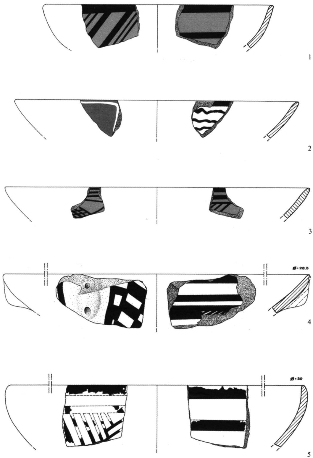
Πίνακας Π.8: 1-5. Γραπτή κεραμική. Στρώμα 3. Κλίμακα 1:2
