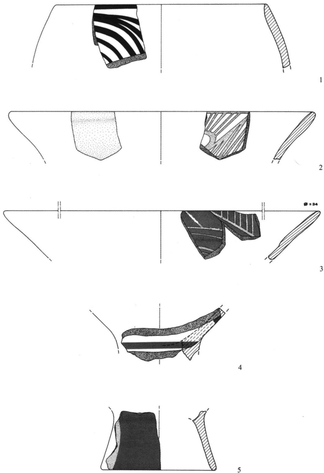
Πίνακας II.26: 1-5. Γραπτή κεραμική. Στρώμα 1. Κλίμακα 1:2
