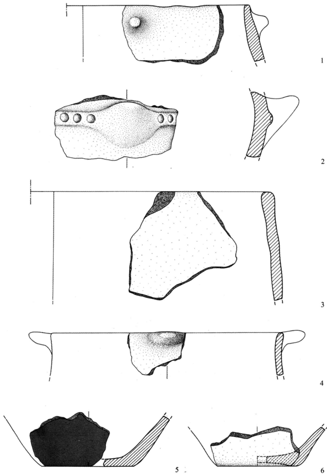
Πίνακας Π.15: 1.3-6. Μονόχρωμη κεραμική, 2. Με ανάγλυφη διακόσμηση. Στρώμα 3. Κλίμακα 1:2
