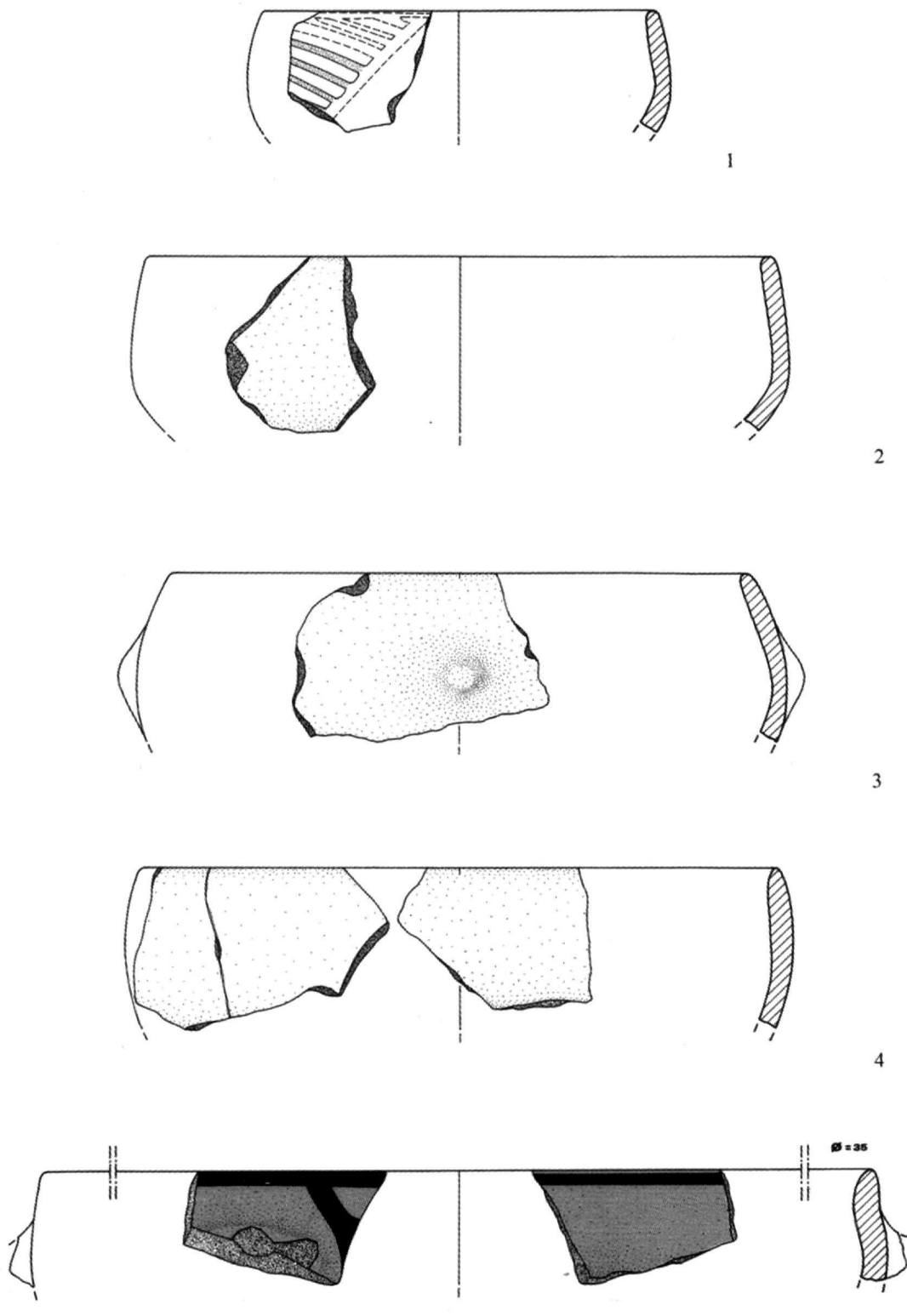
Πίνακας Π.25: 1.5. Γραπτή, 2-4. Μονόχρωμη κεραμική. Στρώμα 1. Κλίμακα 1:2
