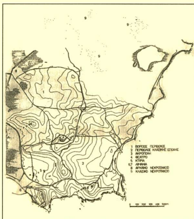
Εικ. 5: Τοπογραφικό σχεδιάγραμμα των Αβδήρων, όπου σημειώνονται οι δύο περιβόλοι της αρχαίας πόλεως (Θράκη, Γενική Γραμματεία Περιφέρειας Ανατολικής Μακεδονίας-Θράκης 1994, 62).
